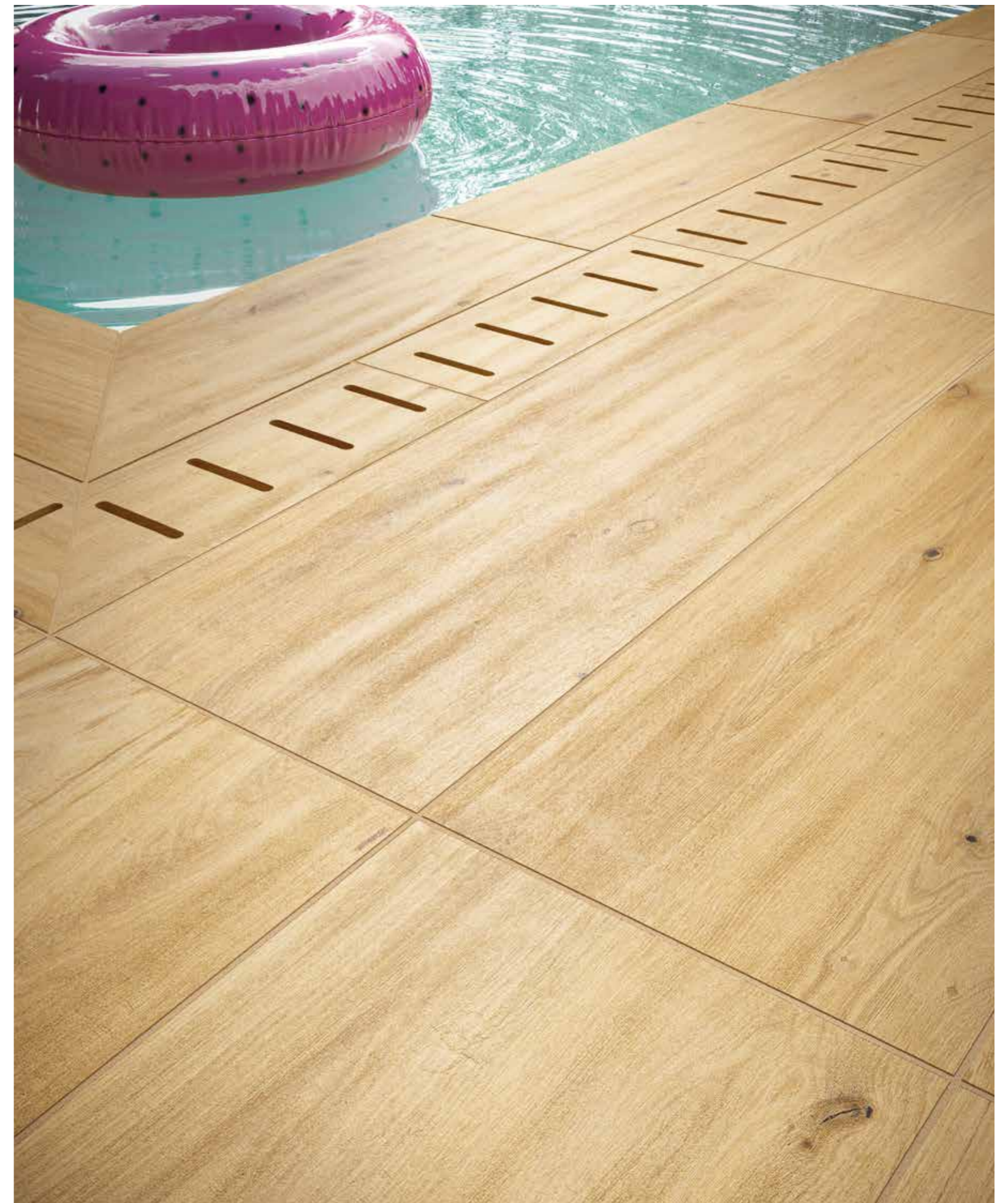
Outdoor_Pavimento . Floor: Thun 40x120 . 16"x48" rettificato - GRIP 20mm / Gradino costa retta 33x120 . 13"x48" rettificato - GRIP 20mm / Angolo Int. Gradino Costa Retta 33x120 . 13"x48" rettificato - GRIP 20mm / Griglia, Angolo Griglia 20x60 . 8"x24" rettificato - GRIP 21mm
